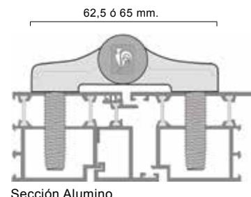
Sección Aluminio
