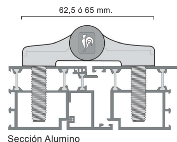
Sección Aluminio
