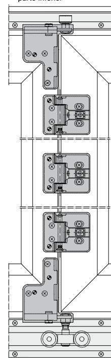
Corte con carros en parte inferior 1 : 2,5
