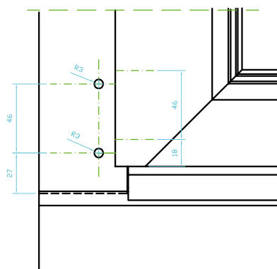
Posición de la bisagra inferior de marco (BIKFMSL) y hoja (BIKFHNSLT)
