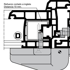
Corte con carros en parte inferior 1 : 2,5
