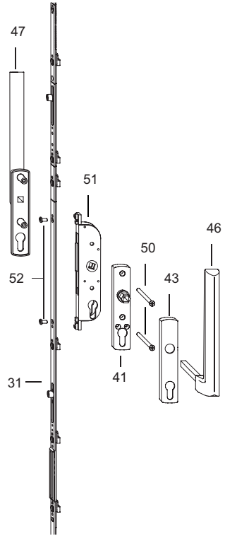
Manilla interior y exterior cerrable Manilla exterior plana
